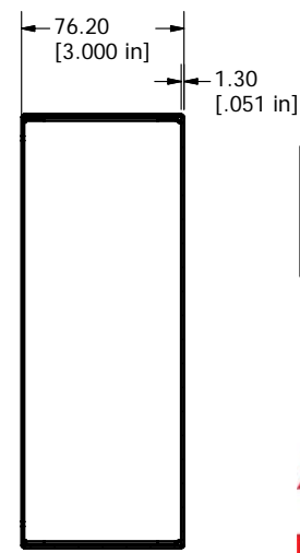
SECTION A-A
